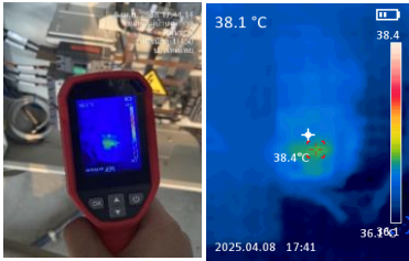
ตรวจสอบความร้อน Breaker inverter 38.1 °C
