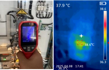
ตรวจสอบความร้อน MCCB 37.9 °C
