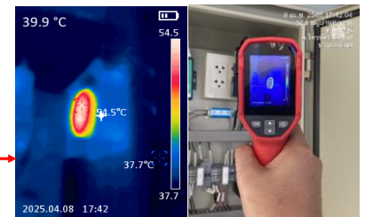
FAN 39.9 °C
