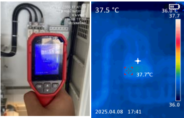
ตรวจสอบความร้อนฟิวส์ MCCB 37.5 °C
